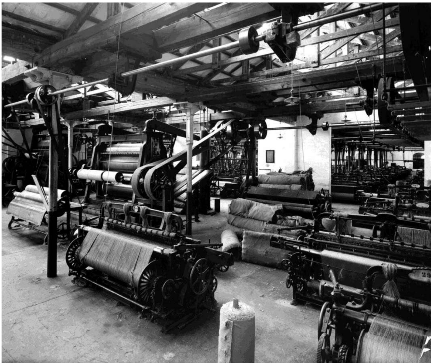
1940-45. Jutificio, sala finissaggio dove la tela veniva stirata facendola passare attraverso i “calandri” (rulli) riscaldati all’interno (collezione Roberta Trevisan).
