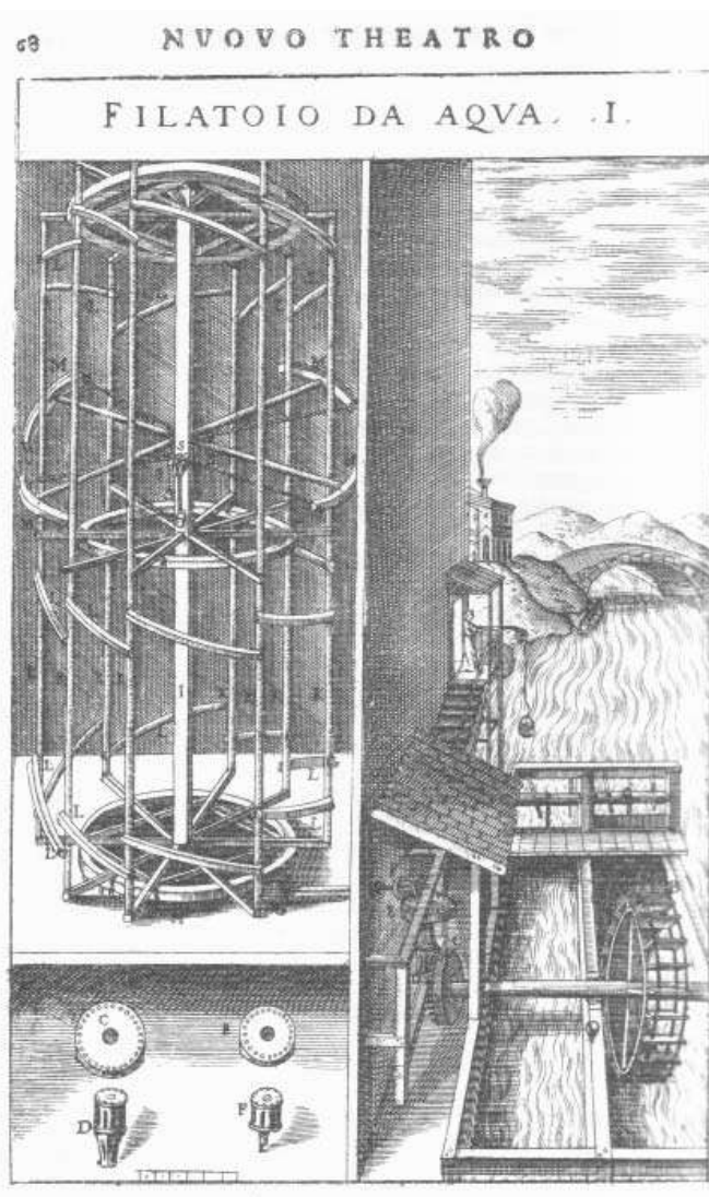
Orsoglio o filatoio alla bolognese (V. Zonca, Novo teatro di macchine et edifici , Padova 1607).
